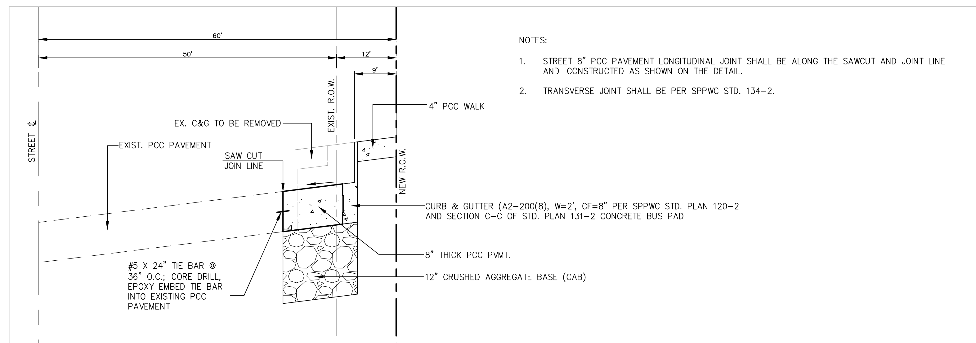
A SECTION SCALE: HORIZ. 1"=10' VER. 1"=1'
